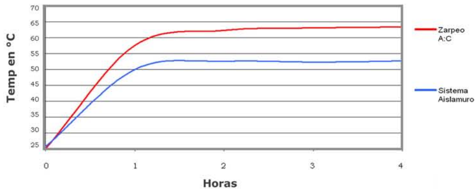
Gráfica de Sistema Aislamuro vs Zarpeo Convencional de arena : cemento a 1" de espesor
